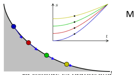
La cicloide es tautócrona
