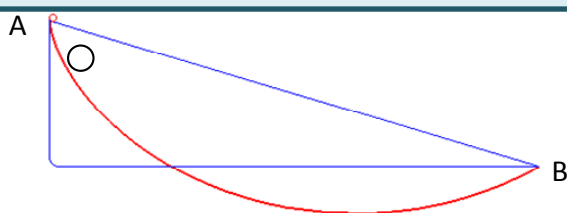
La cicloide es braquistócrona
