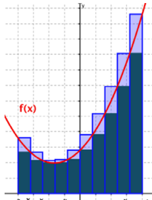
Suma inferior y superior con la partición P_2
